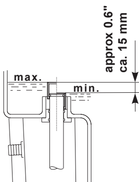
ÖWAMAT 2
