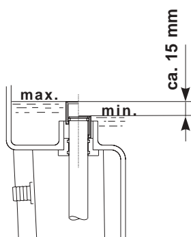
ÖWAMAT 2
